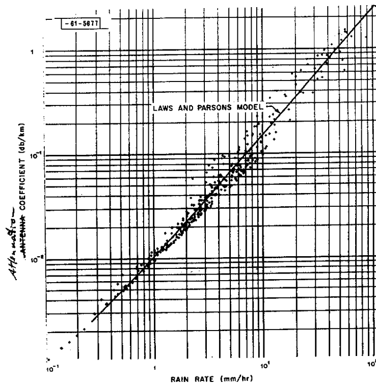
(d) Frequency: 9.35 GHz.
