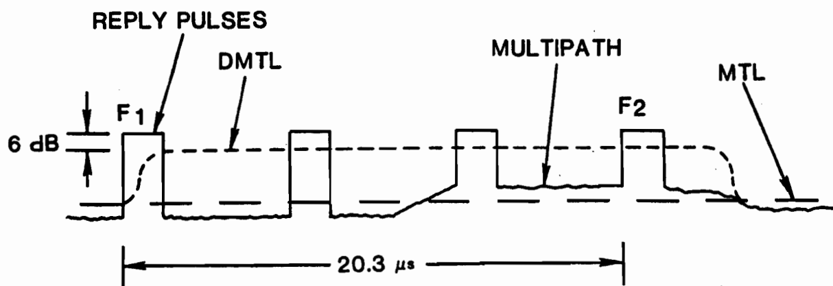
Fig. 3-27. Dynamic MTL.
