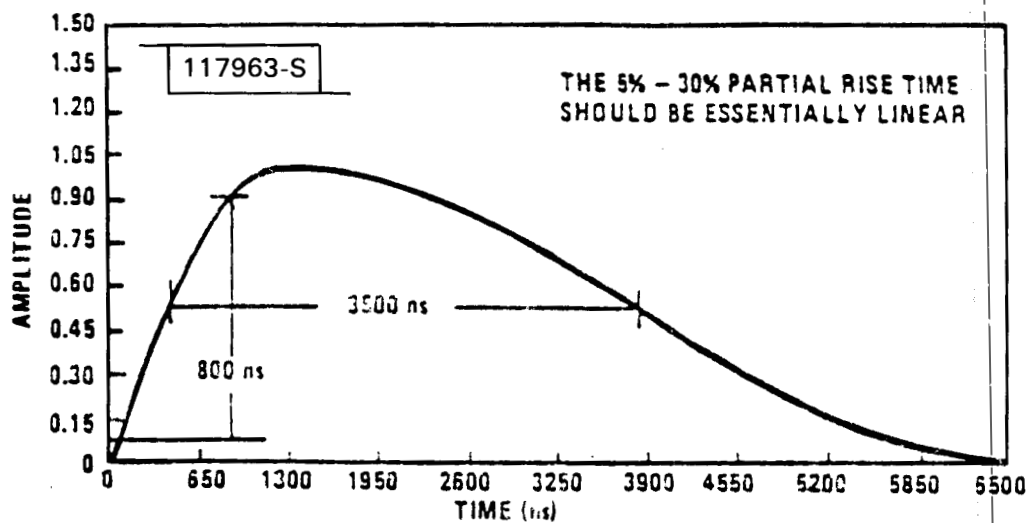
Fig.2-2. DME/P cos-cos 2 waveform.
