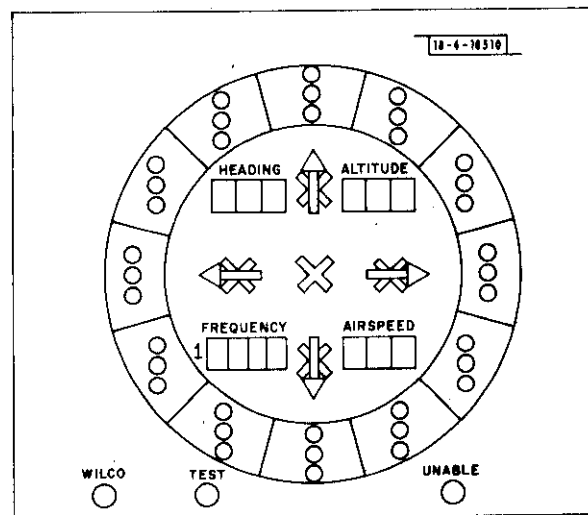
Fig. 4-7. IPC/PWI/ATC Display
