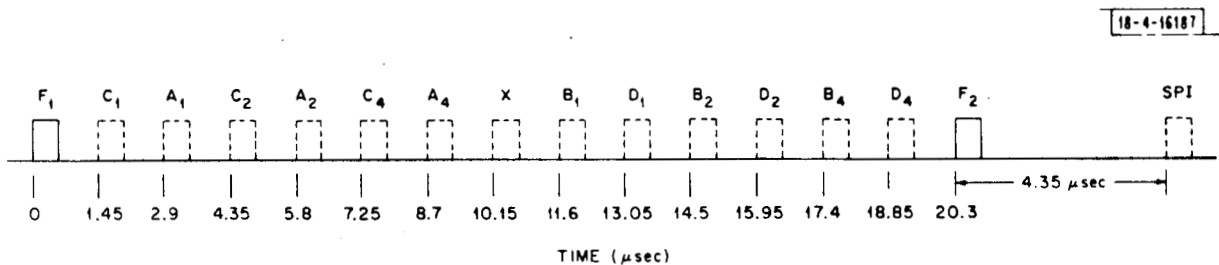
Fig. 3.3-1. ATCRBS reply format.
